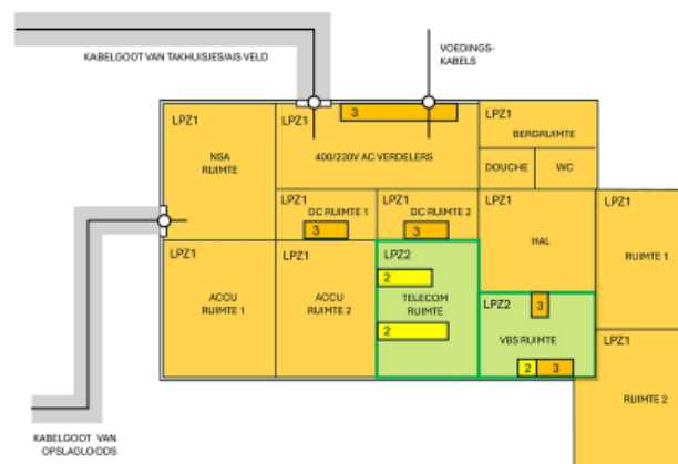
EM zonering CDG conform TenneT eisen
