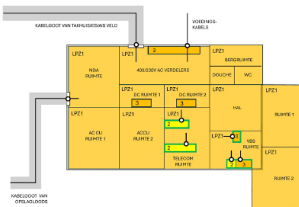
EM zonering CDG conform zoals uitgevoerd
